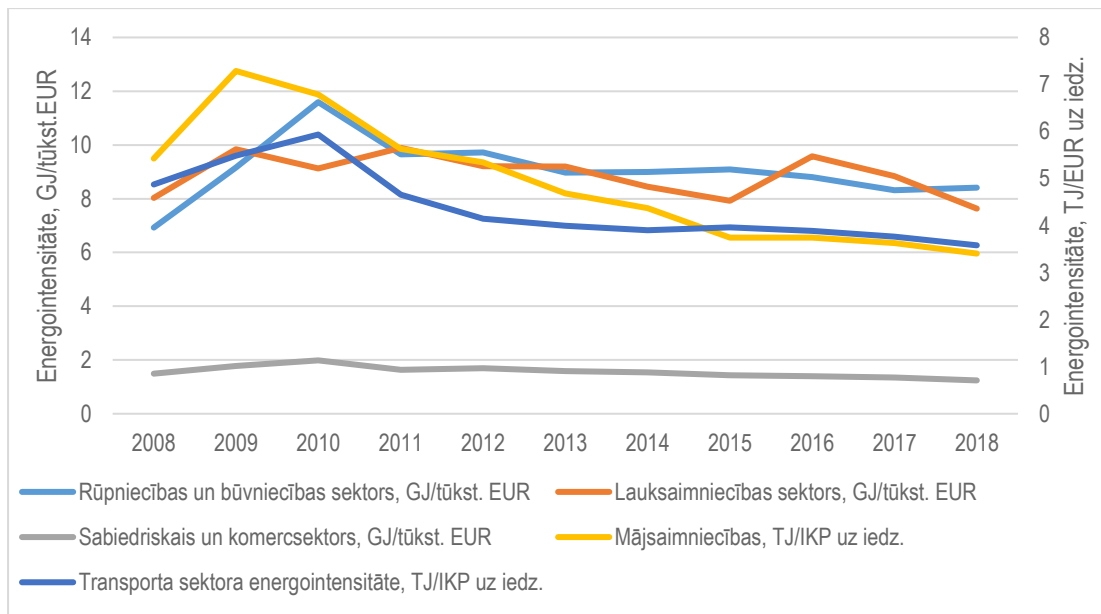
Attēls 2.8 Sektoru energointensitātes salīdzinājums
